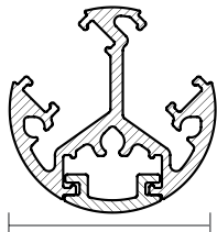
Kulmatolppa 90°
