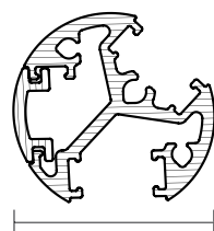
Kulmatolppa 135°
