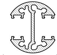
Keskitolppa
